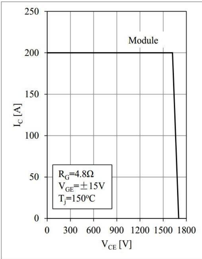
Fig 5. RBSOA
